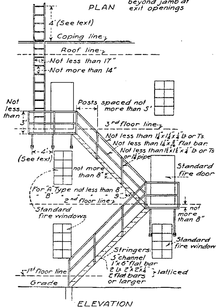
FIRE ESCAPES
